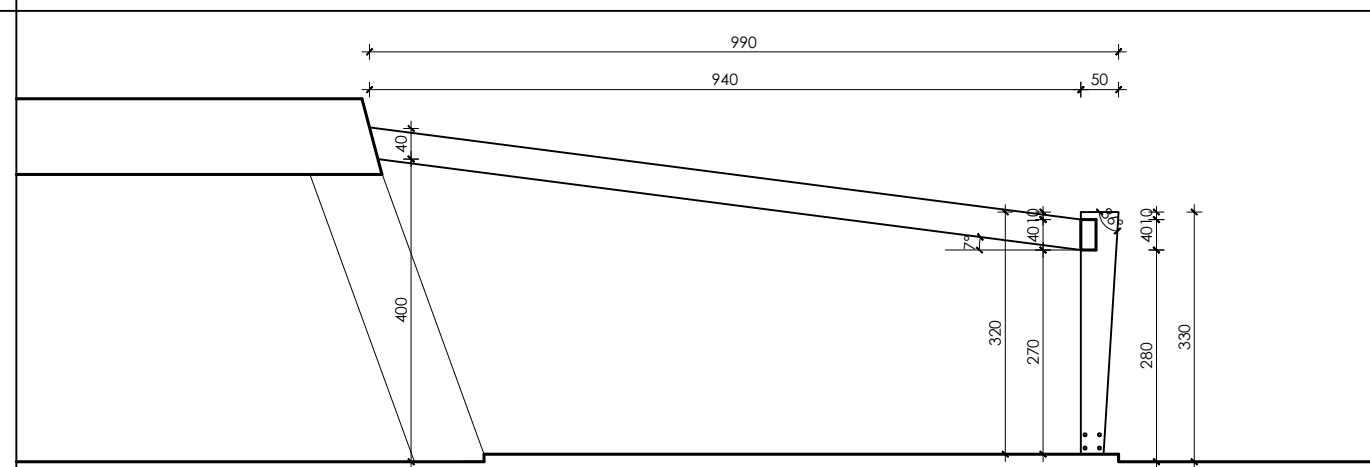
PRESJEK
