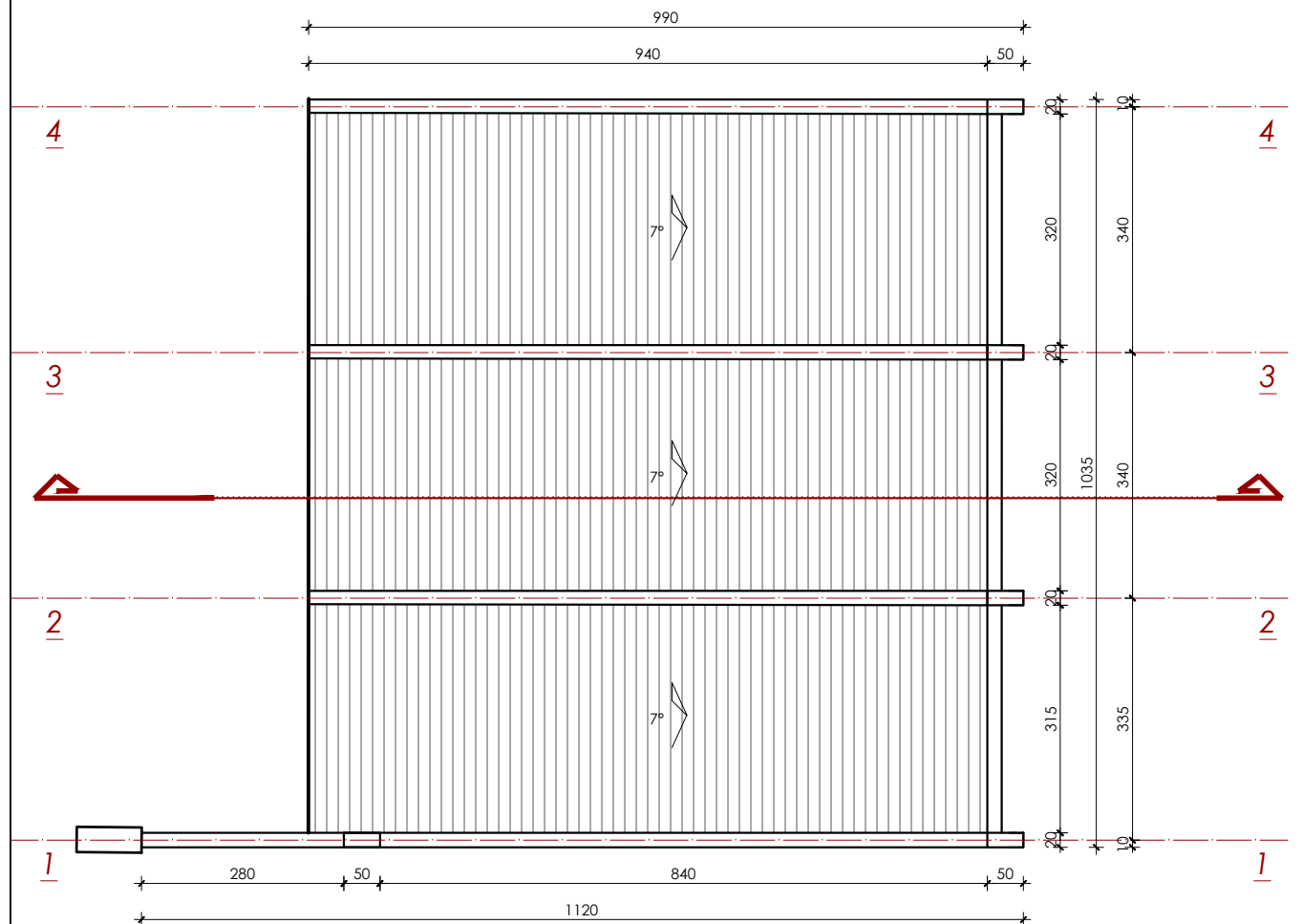
OSNOVA KROVA
